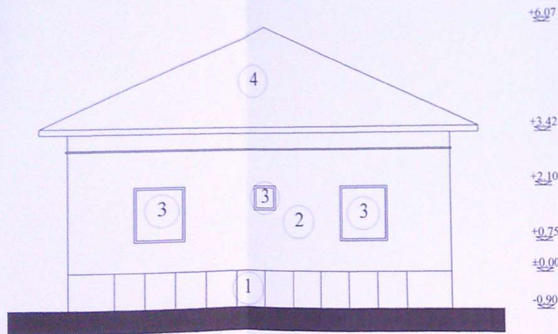
FATADA EST
